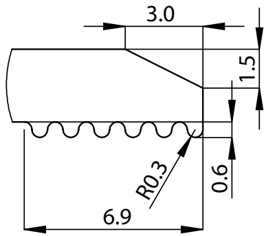
Einzelheit A Maßstab 4:1
